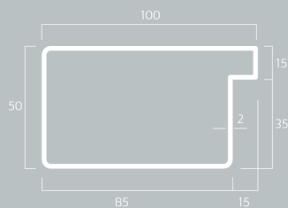
16D Kg/m 4,65
