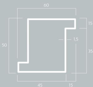
16Z Kg/m 2,56
