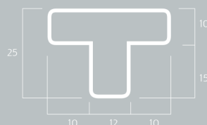
10B Kg/m 1,40
