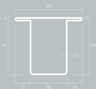
SF2B Kg/m 2,52
