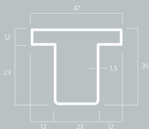
2B Kg/m 1,88
