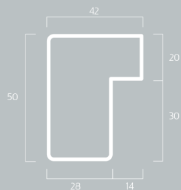
SFG2 Kg/m 2,16
