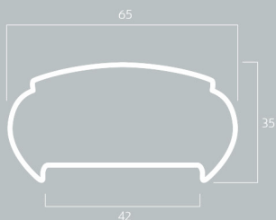
MT7-15/10=Kg/ml 2,15
