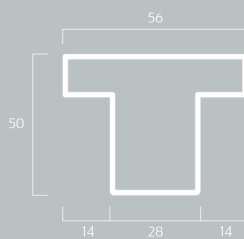
SFG4 Kg/m 2,50
