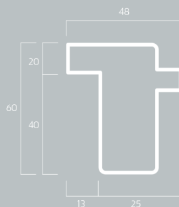
SFG9 Kg/m 2,52
