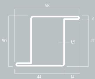
SF3B Kg/m 2,52
