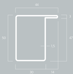
SF1B Kg/m 2,15
