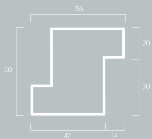
SFG6 Kg/m 2,50
