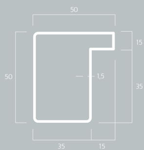
16A Kg/m 2,33
