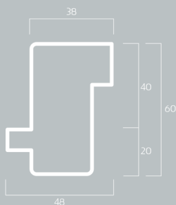
SFG10 Kg/m 2,52
