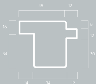
SFG11 Kg/m 2,61
