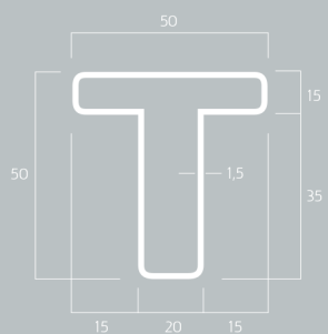
16B Kg/m 2,33
