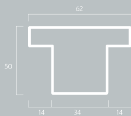
SFG3 Kg/m 2,52
