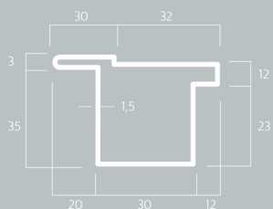
2T Kg/m 2,30
