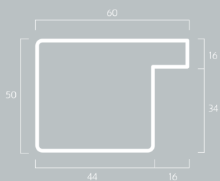
SFG1 Kg/m 2,52
