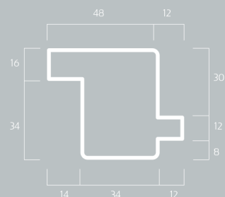
SFG12 Kg/m 2,61
