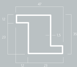
2Z Kg/m 1,88
