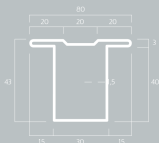
15T Kg/m 2,45
